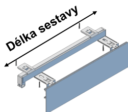
Sestavy typ C záclona nebo závěs + krycí čelo typ 53 Elegant
